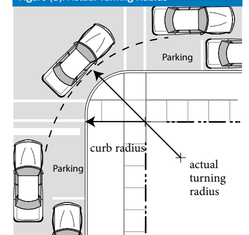
Figure (8). Actual Turning Radius
